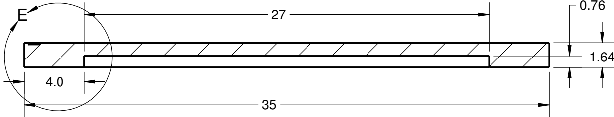
SECTION B-B SCALE 4 : 1
